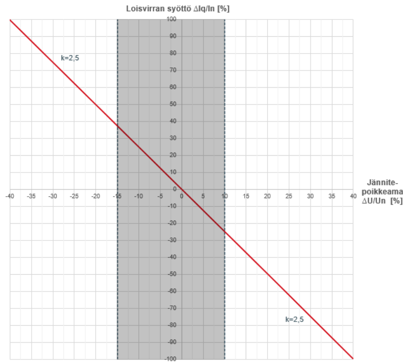
• Kuva 10.3. Loisivirran aktivointirajat jännitteen perusteella sekä k-kertoimen määrittely. Loisivirran syöttö aktivoituu harmaan alueen ulkopuolella. Nuolen alkupiste kuvaa loisivirransyötön aktivoitumista ja suunta lisäloisivirran kasvua jännitepoikkeaman kasvaessa. Suora viiva kuvaa kulmakertoimta k=2,5 .
