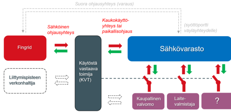
Kuva 10.4. Sähkövaraston ohjaus ja kaukokäyttö. Sähkövaraston käytöstä vastaava toimija operoi sähkövarastoa. Fingrid voi antaa sähkövarastolle ohjauksia (punaiset nuolet) sekä vastaanottaa tilatietoja (vihreät nuolet) sähköisellä ohjausyhteydellä. Erillisen, suoran Fingridin ja sähkövaraston välisen ohjausyhteyden toteuttamisesta päätetään erikseen. Käytöstä vastaavalla toimijalla voi lisäksi sähköinen ohjausyhteys (katkoviivanuolet ylhäällä) tai muuta tiedenvaihtoa mahdollisen liittymispisteen verkkohaltijan (esim. jakeluverkko-yhtiö) tai muiden sähkövarastoa mahdollisesti ohjaamaan kykenevien toimijoiden kanssa (katkoviivanuolet alhaalla). Käytöstä vastaavalla toimijalla on mahdollisuus oikeuttaa ja rajoittaa muiden toimijoiden ohjauskykyä.
