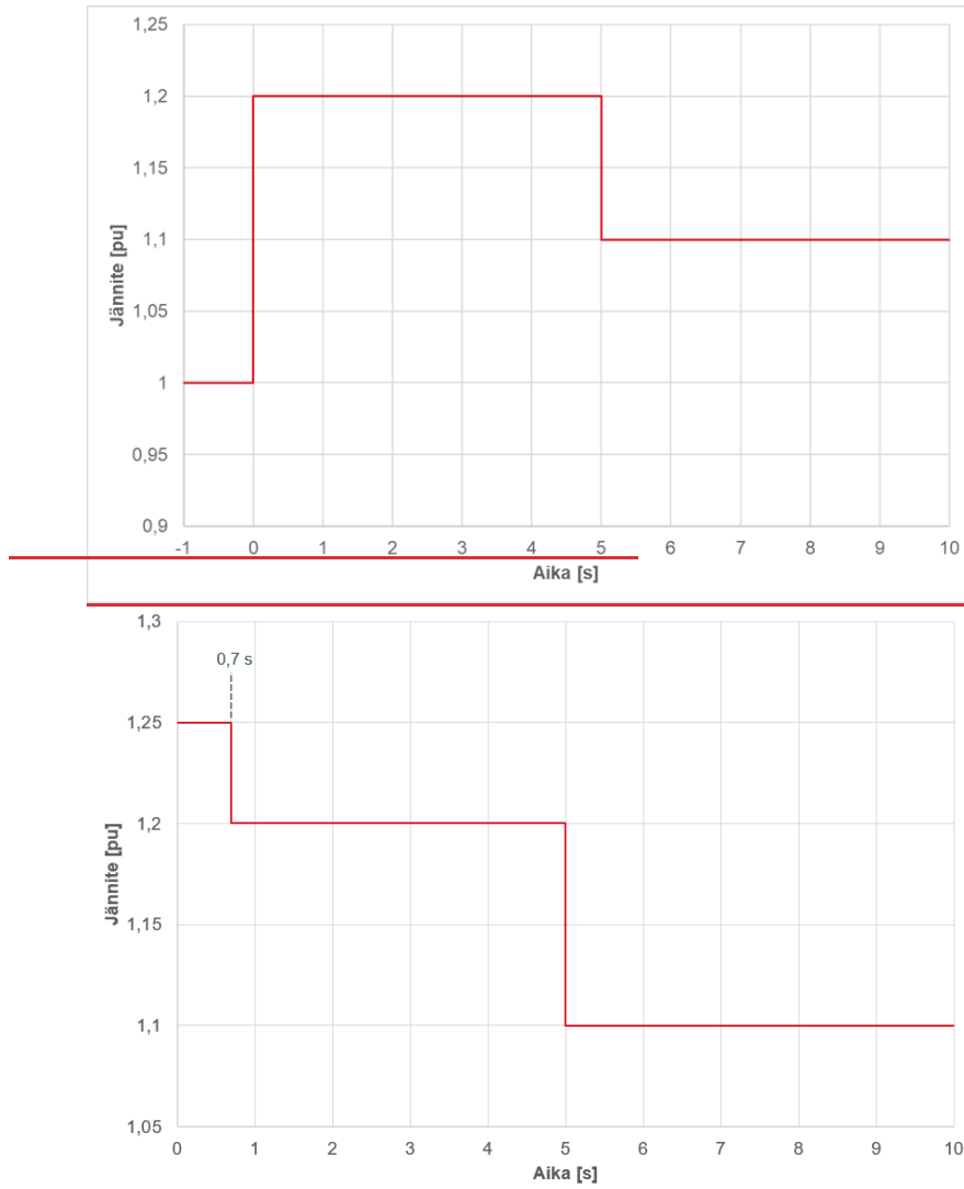
Kuva 10.2. Lyhytaikaista ylijännitettä vastaava liittymispisteen pääjännite, jonka aikana ja jälkeen tyyppin B, C ja D sähkövarastojen tulee jatkaa toimintaansa normaalisti. Jännitteen suhteellisarvo 1,0 pu on liittymispisteen normaali käyttöjännite ennen häiriötä.
